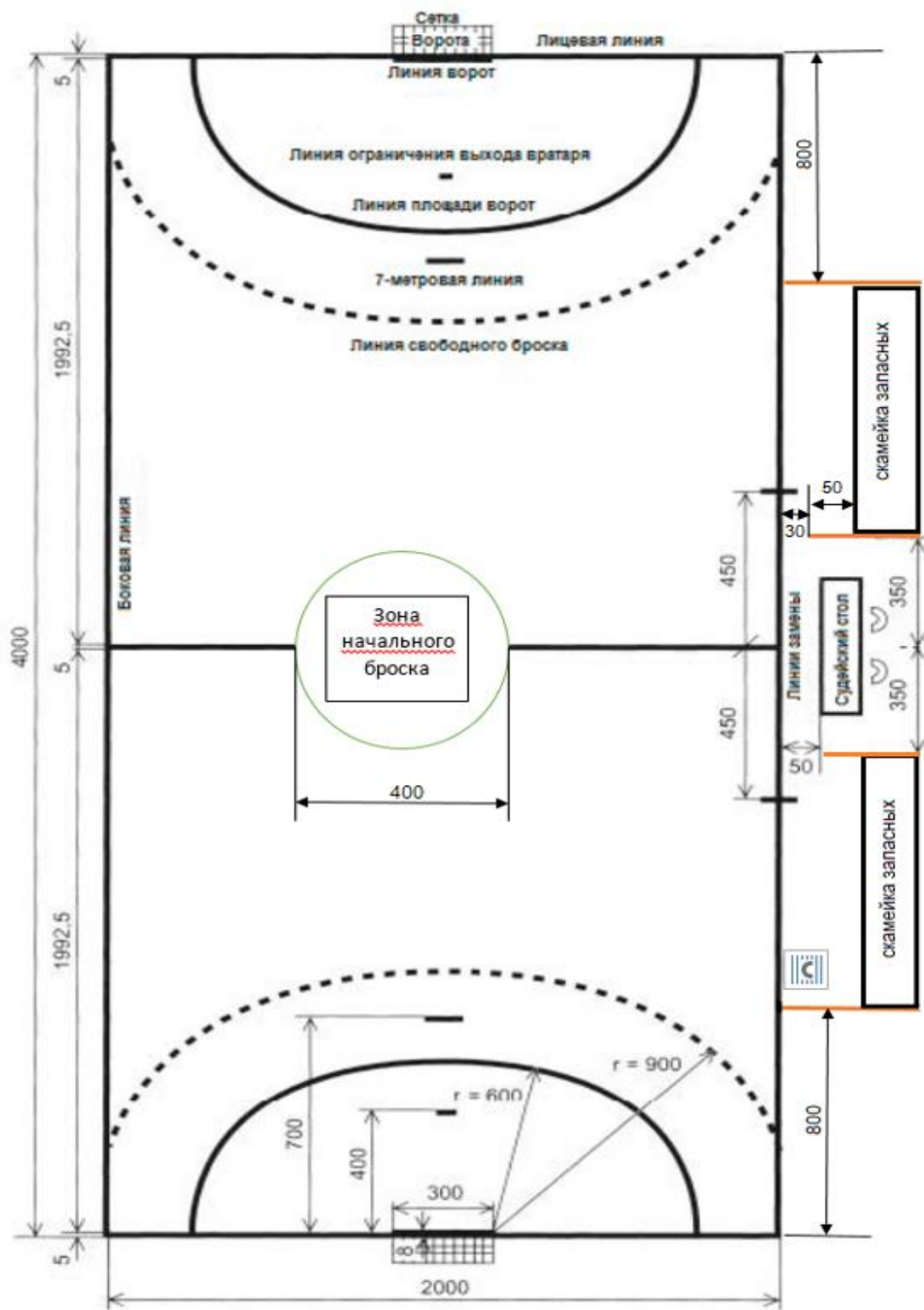
Рисунок 1. Игровая площадка (размеры – в см).
