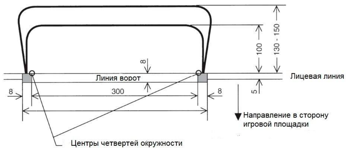
Рисунок 2а. Ворота
