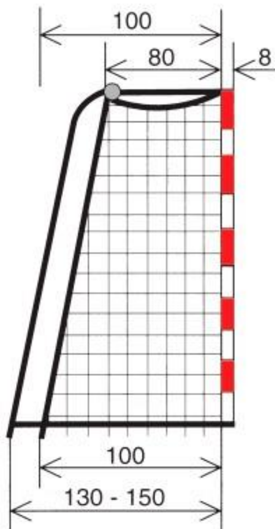
Рисунок 2в. Ворота. Вид сбоку.
